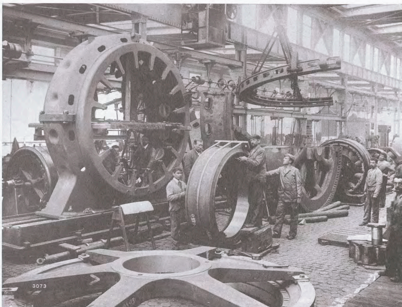
Generatorenbau bei Brown Boveri in Baden, 1897.
